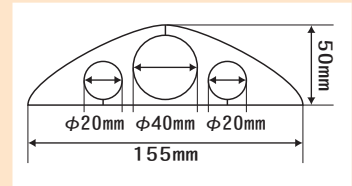
69-3-40 φ40mm×4m
