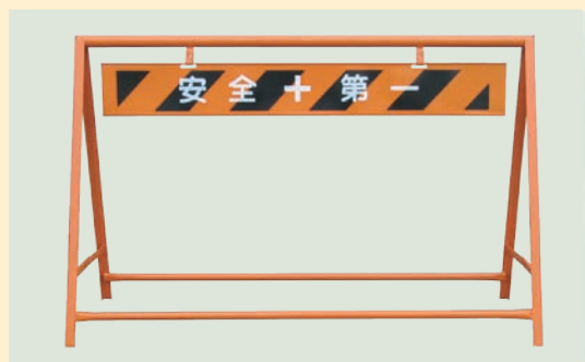
40-2 A型バリケード(オレンジ) ●1200Aバリ大: W1200×H800mm 重さ: 約 4.0kg ●900Aバリ小: W900×H800mm 重さ: 約 3.6kg
