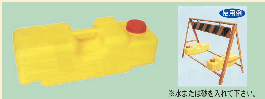
40-9 バリブロック ●W500×D170×H170mm ●材質: HDPE ●重量: 満水時約12kg
