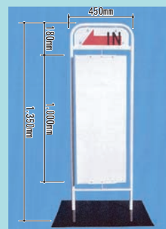
●板面：アルミ複合板 3t
